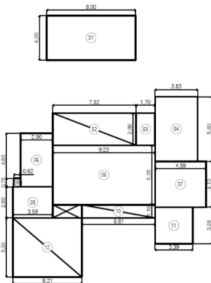
PLANTA DE SUPERFICIES ESC. 1:200
